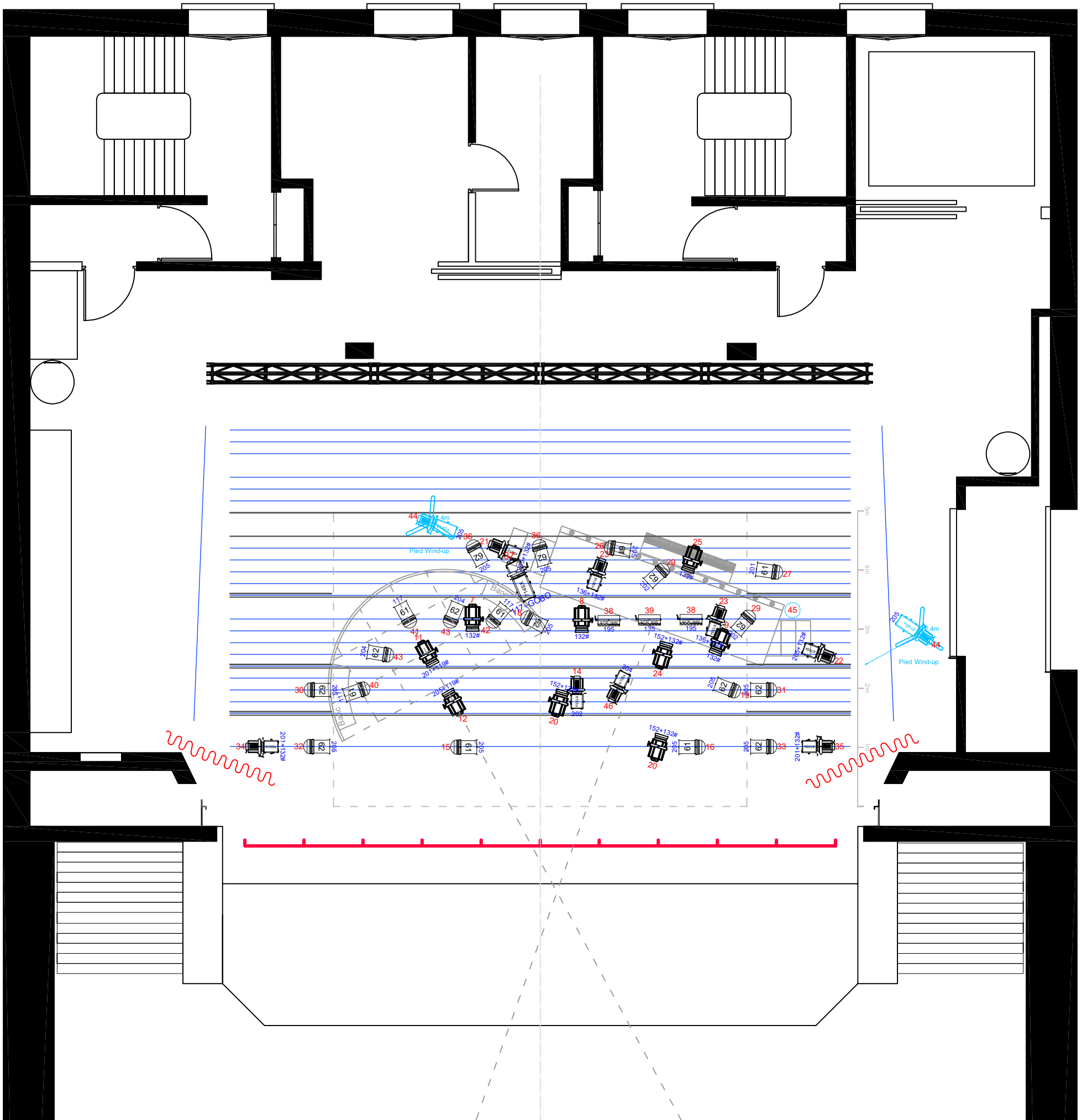
Plan d'implantation spectacle "Maurice et la Miss" Théâtre Armande Béjart - Asnière - Création - A4-1/100e
